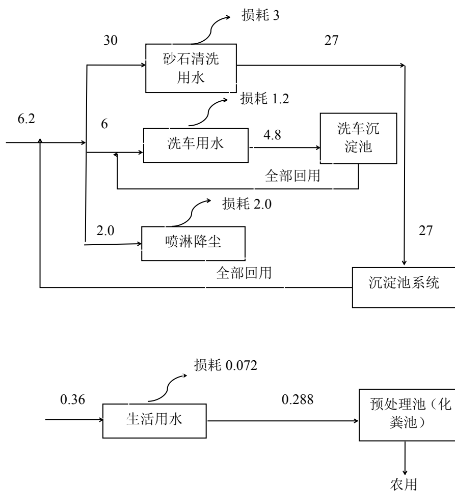
图 2-1 项目水平衡图 单位：m 3 /d
