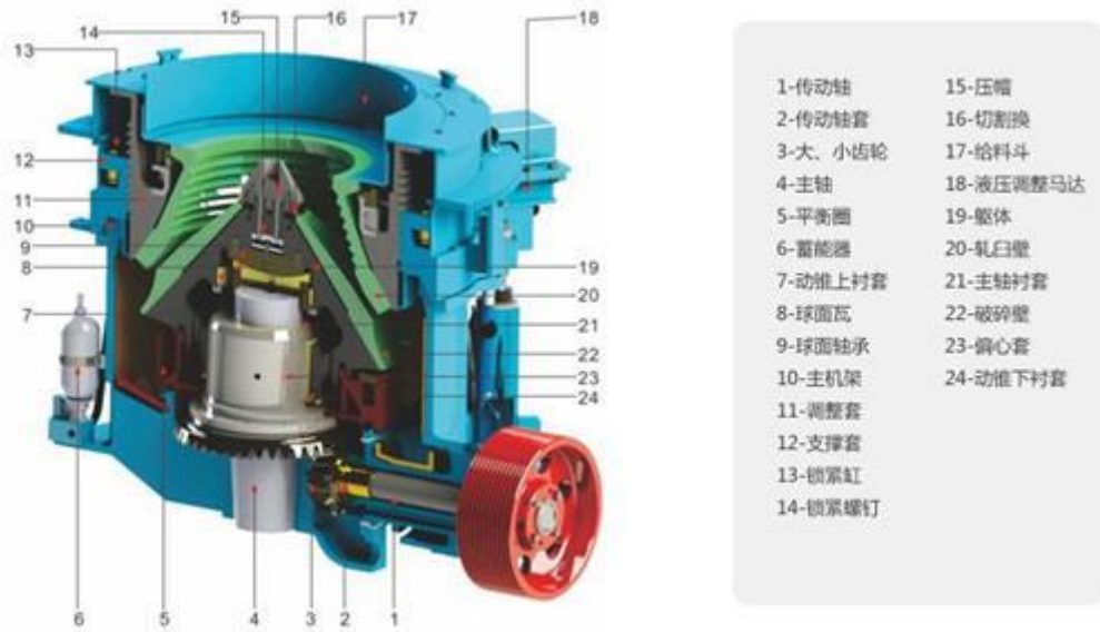
图 2-5 圆锥破碎机工作原理图
