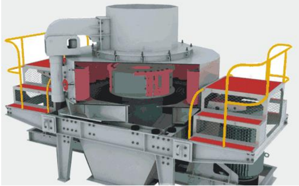
图 2-6 制砂机工作原理图
