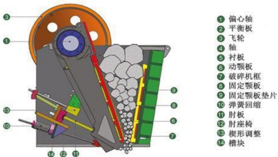
图 2-4 颚式破碎机工作原理图
