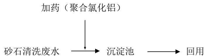
图 4-1 洗砂废水处理工艺流程图
