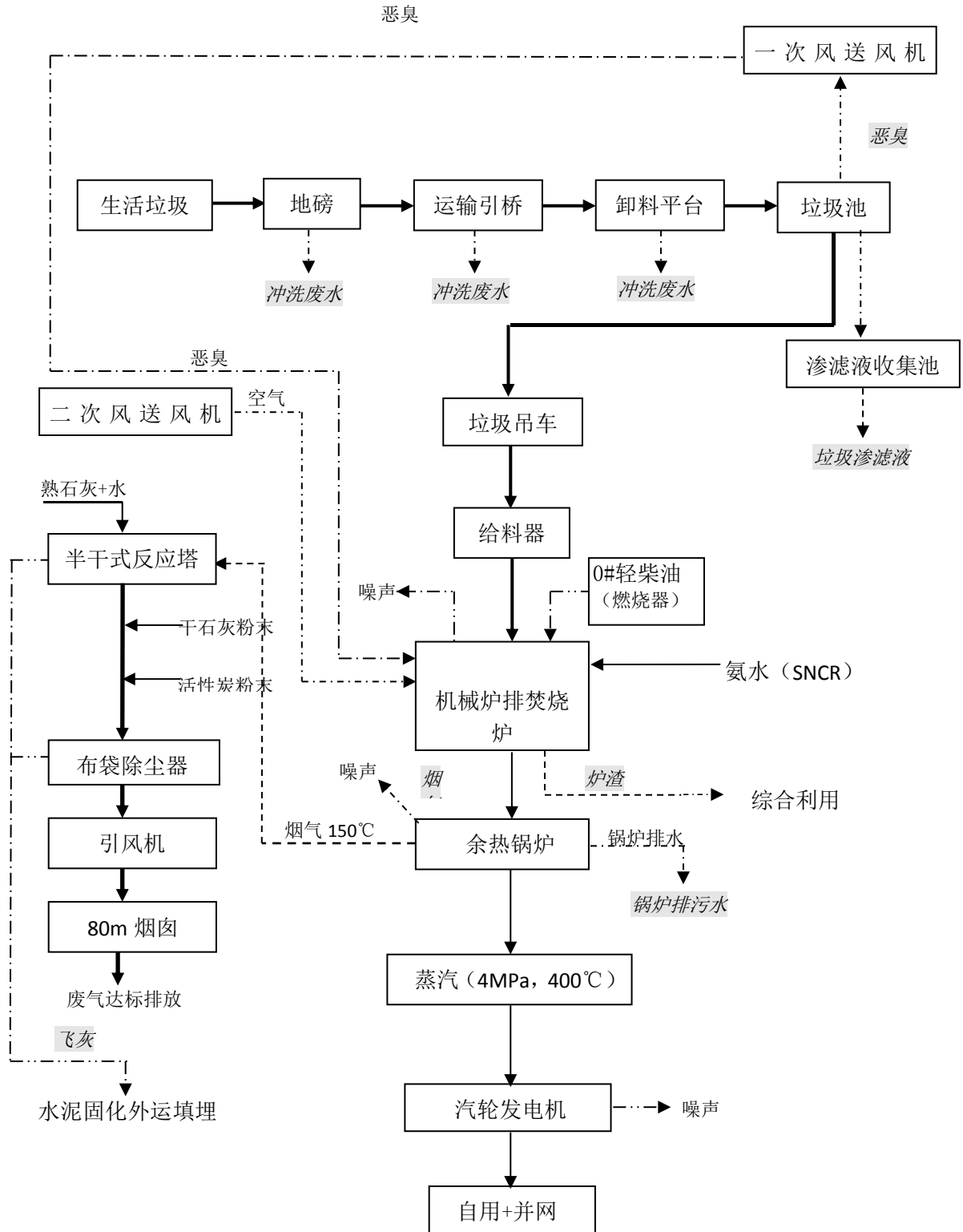
焚烧发电工艺流程及产污环节示意图
